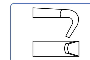
Escuadra con despalme tipo TRA's
